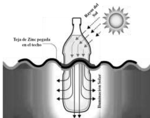
Figura 7: Fijación de la botella al techo de la casa
