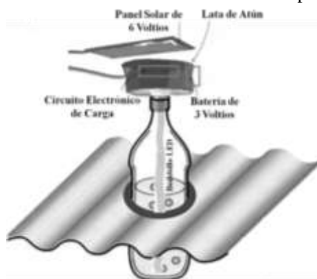
Figura 8: Instalación bombilla nocturna con panel solar
