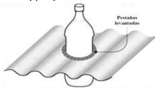
Figura 4: Ubicación y pre-fijación de la botella a la lámina con el dentado
